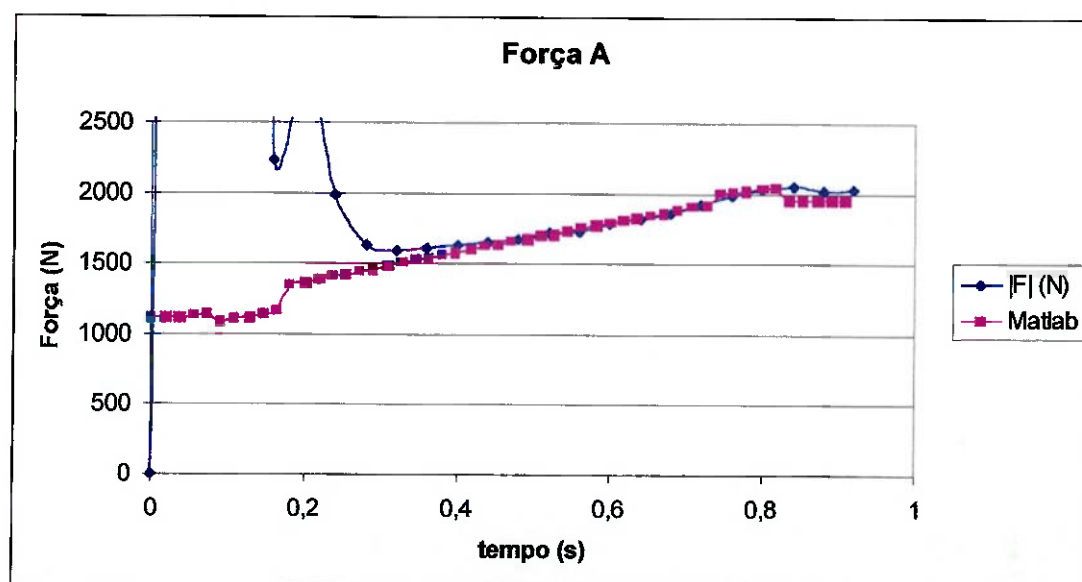
Fig. 9.1 : Gráfico de forças no atuador A
