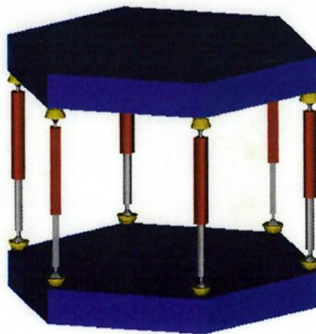
Fig. 2.1 : Estrutura paralela
