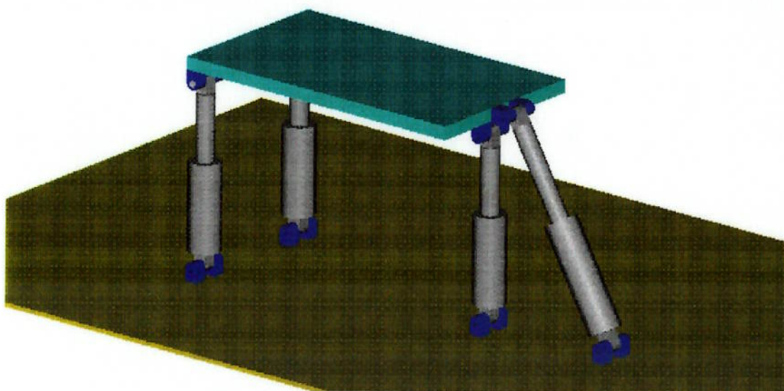
Fig. 4.1 : Plataforma selecionada para projeto
